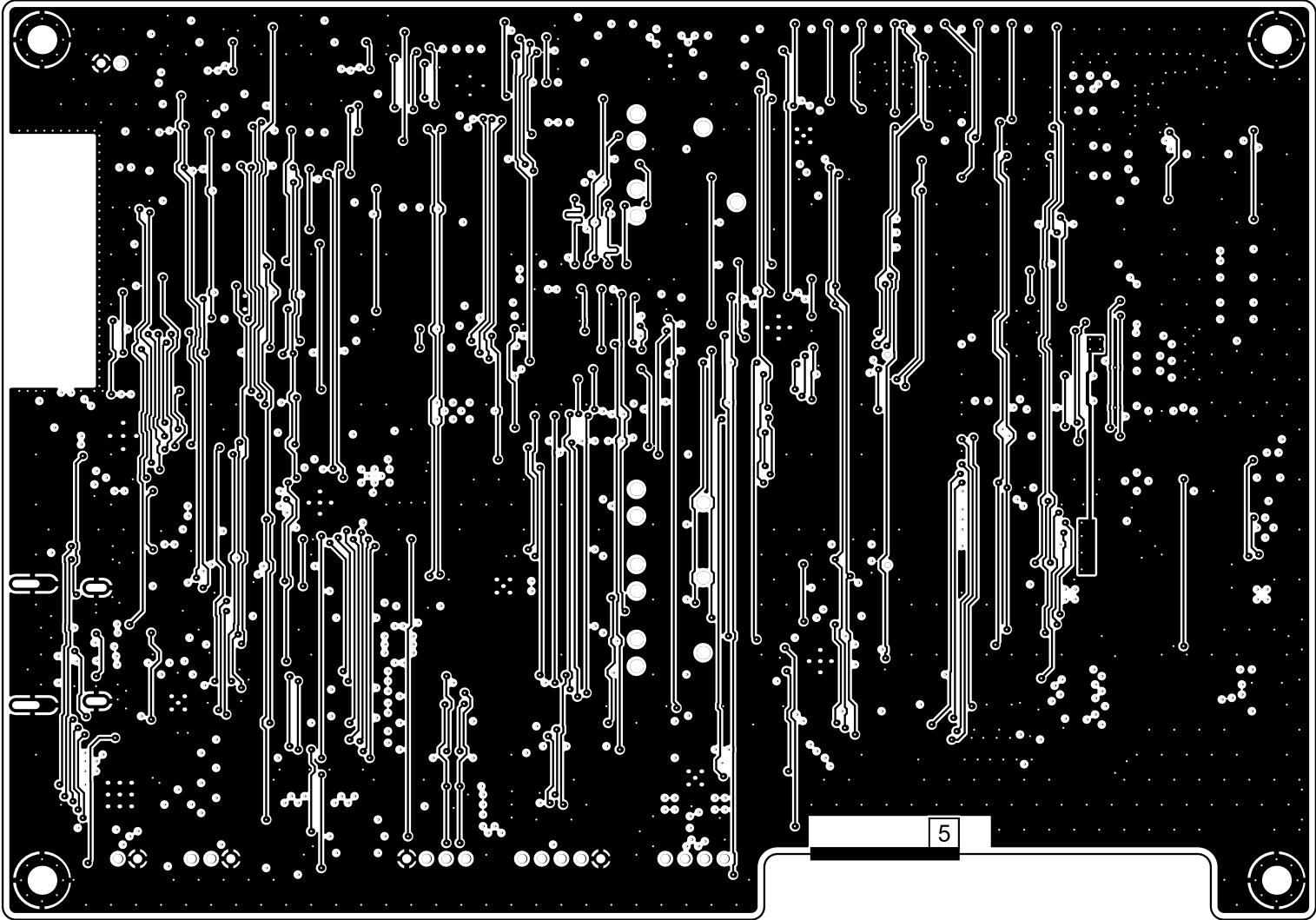
5-SIG-VERT (Scale: 2:1)
