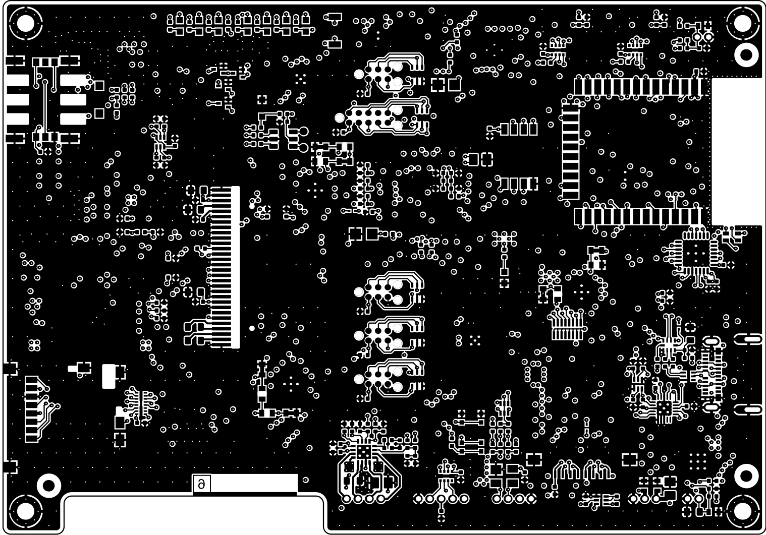
6-GND-BOT (Scale: 2:1)
