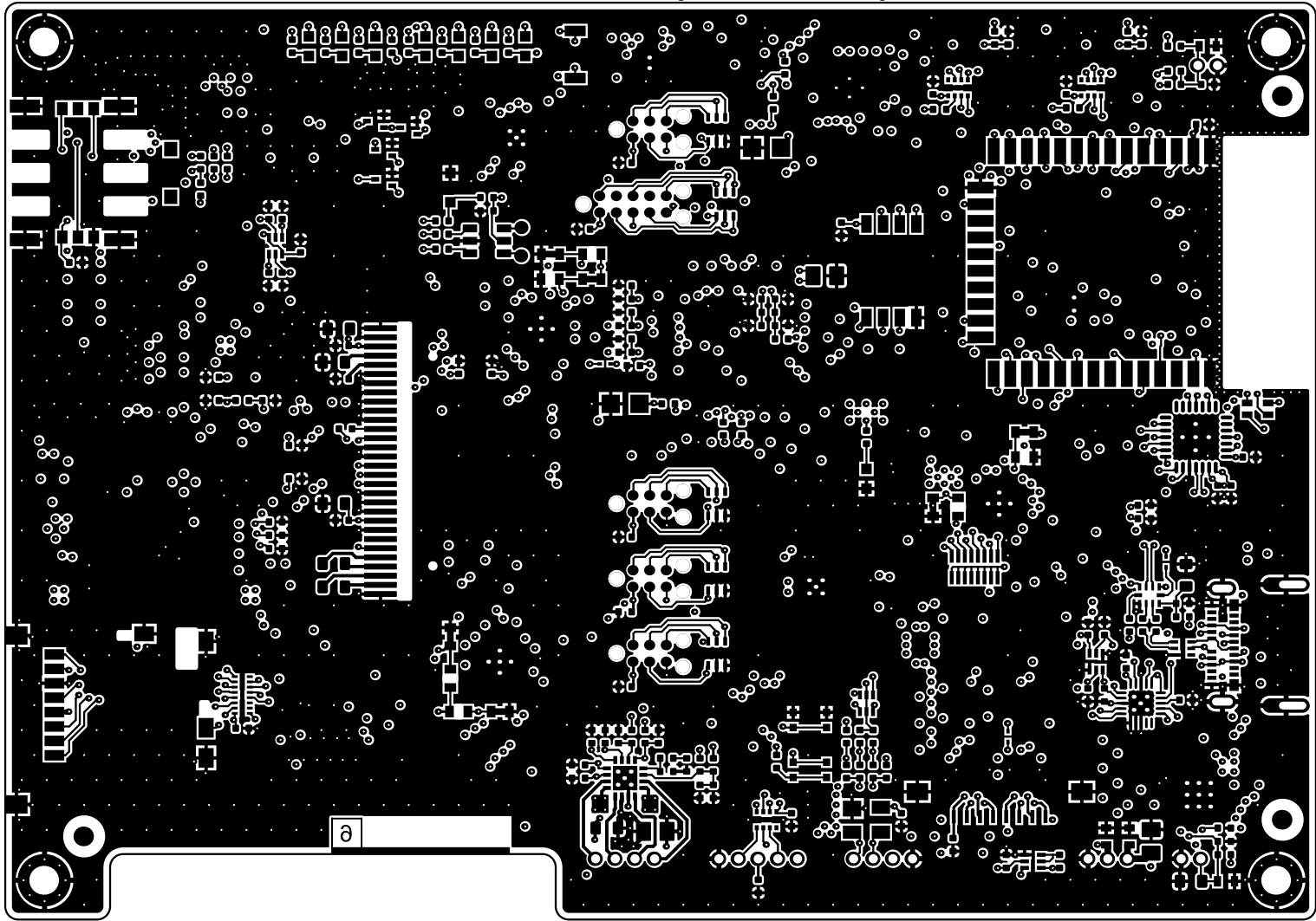
6-GND-BOT (Scale: 2:1)
