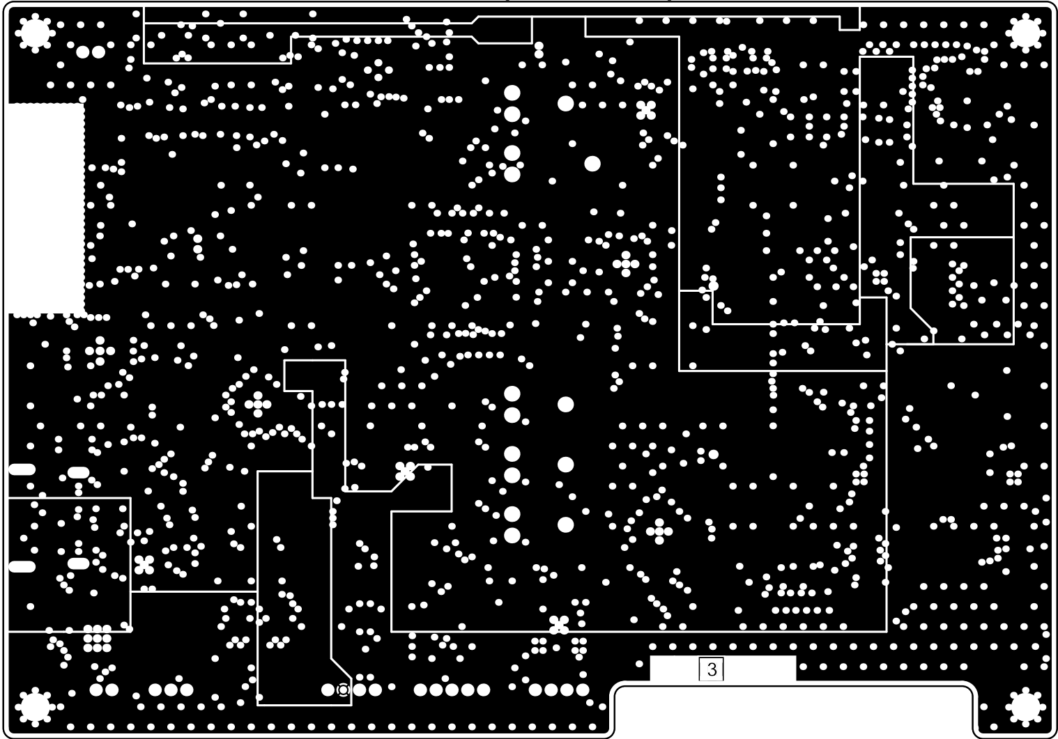
3-PWR (Scale: 2:1)
