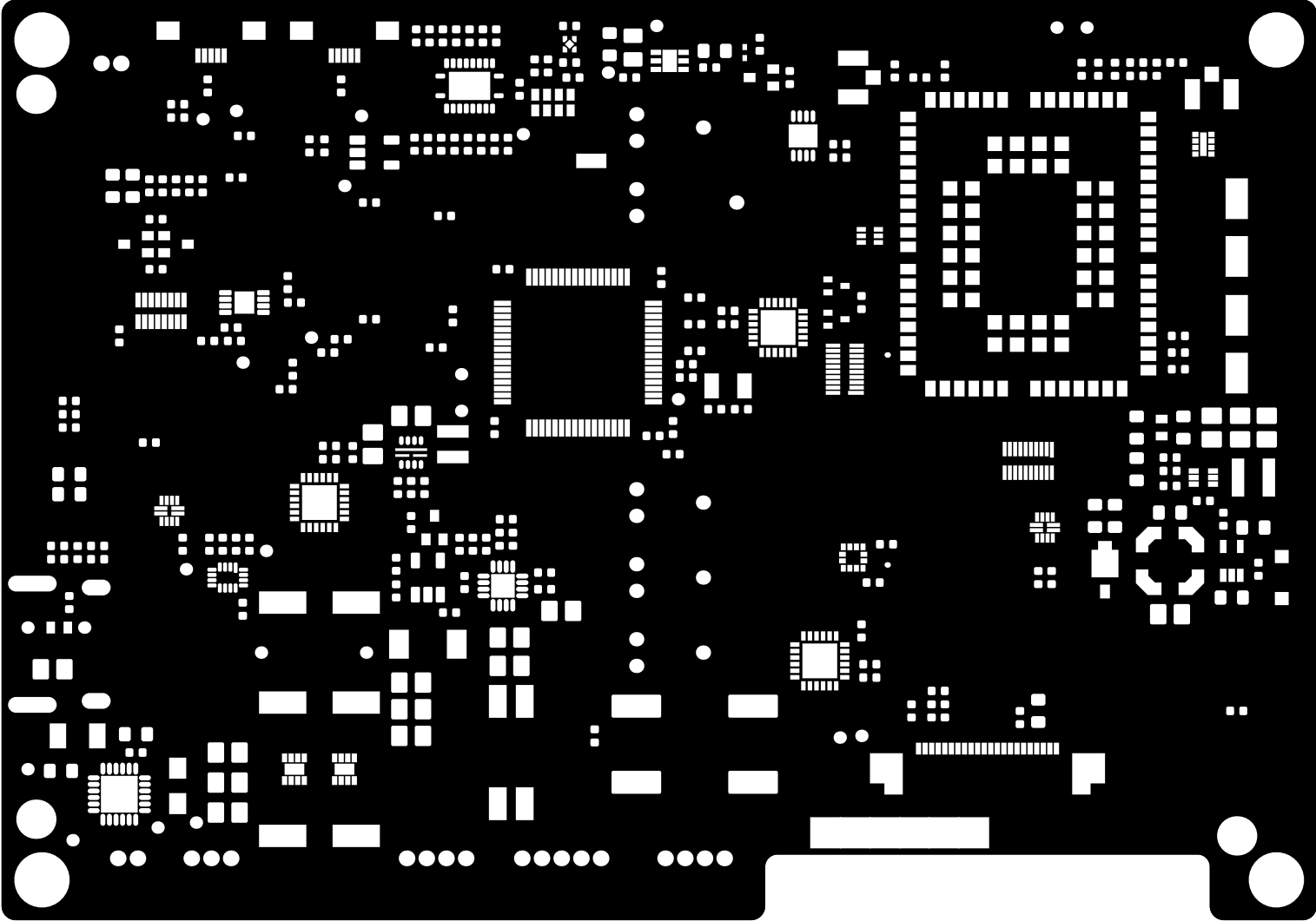
Top Solder (Scale: 2:1)
