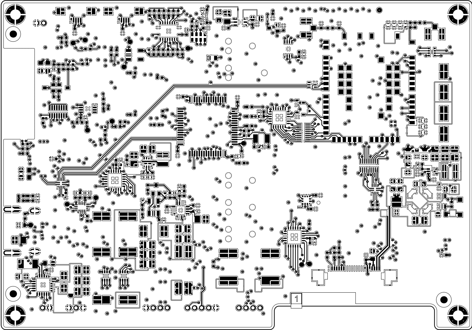
1-SIG-TOP (Scale: 2:1)
