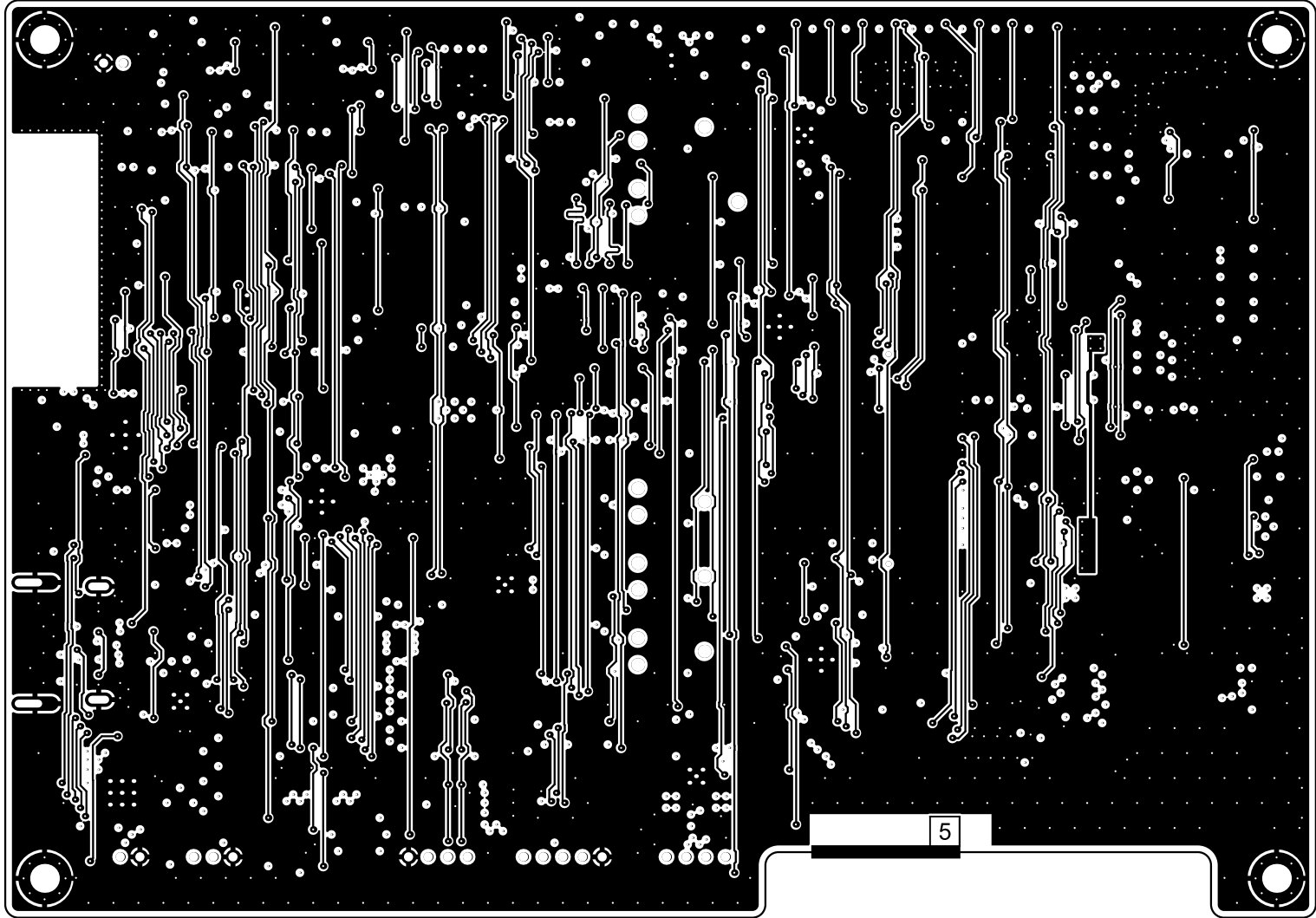
5-SIG-VERT (Scale: 2:1)
