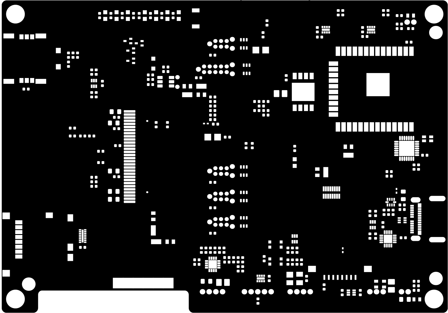
Bottom Solder (Scale: 2:1)
