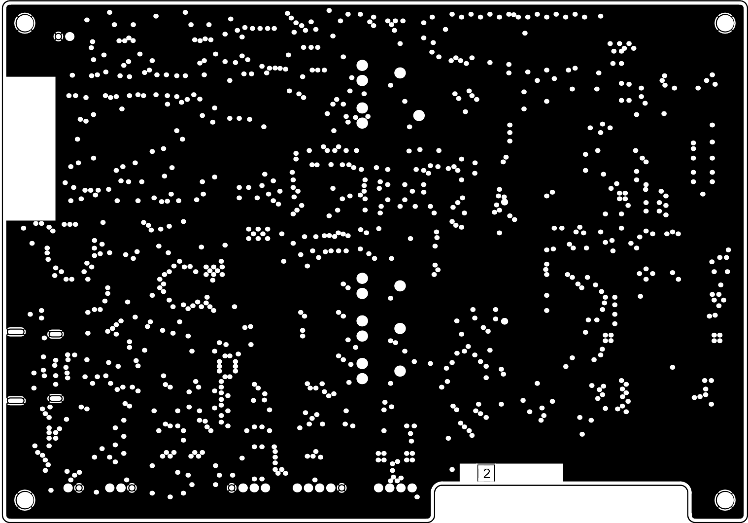
2-GND (Scale: 2:1)
